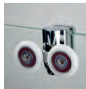
Puertas con rodamientos ajustables en altura. Freno con bloqueo de puerta.
